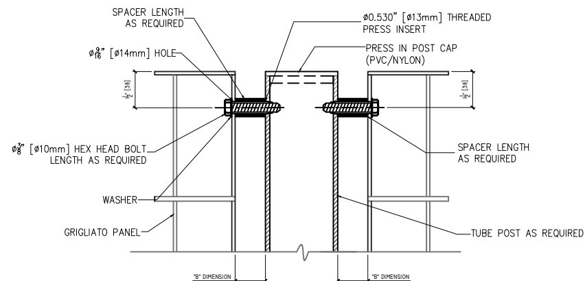
1 GRIGLIATO SPACER CONNECTION DETAIL GA-8 SCALE: N.T.S.
