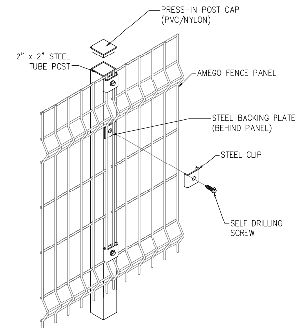
3 CONNECTION DETAIL ISOMETRIC SK1 SCALE: N.T.S.
