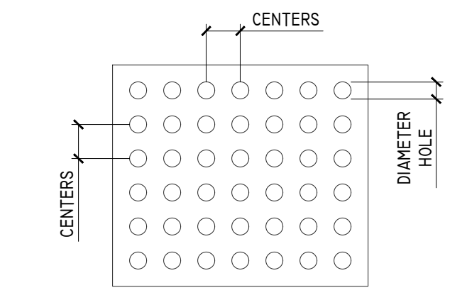
2 STANDARD ROUND HOLES AI SCALE: 3"=1'-0"
