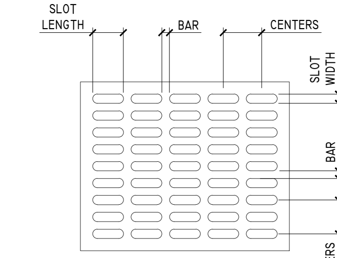
6 STANDARD SLOTTED HOLES AI SCALE: 3"=1'-0"
