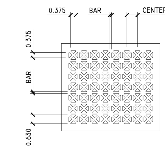
9 GRECIAN DECORATIVE AI SCALE: 3"=1'-0"
