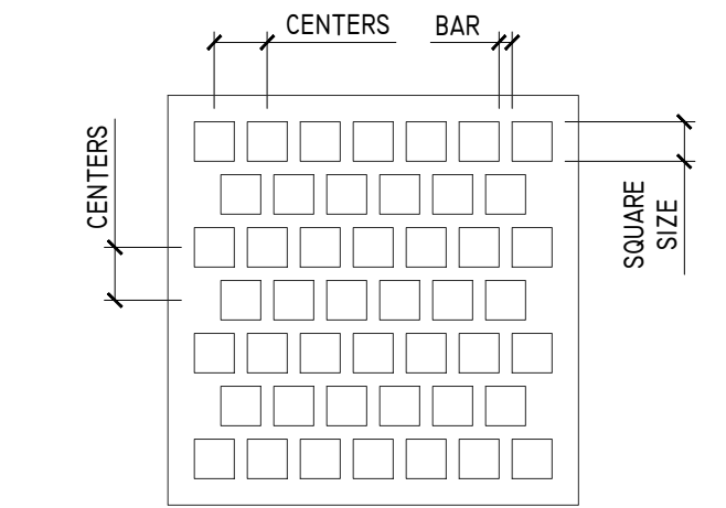
5 STAGGERED SQUARE HOLES AI SCALE: 3"=1'-0"
