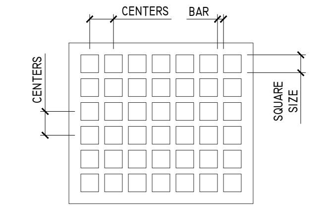
4 STANDARD SQUARE HOLES AI SCALE: 3"=1'-0"
