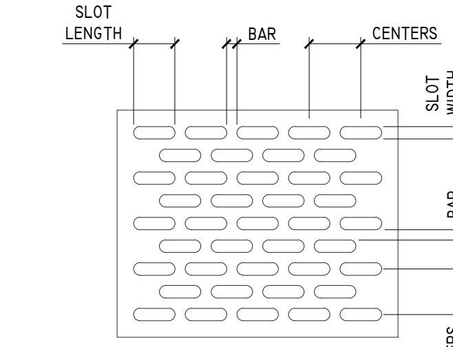
7 STAGGERED SLOTTED HOLES AI SCALE: 3"=1'-0"
