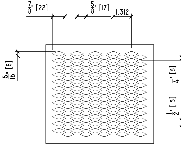
11 DIAMOND STAGGERED DECORATIVE AI SCALE: 3"=1'-0"
