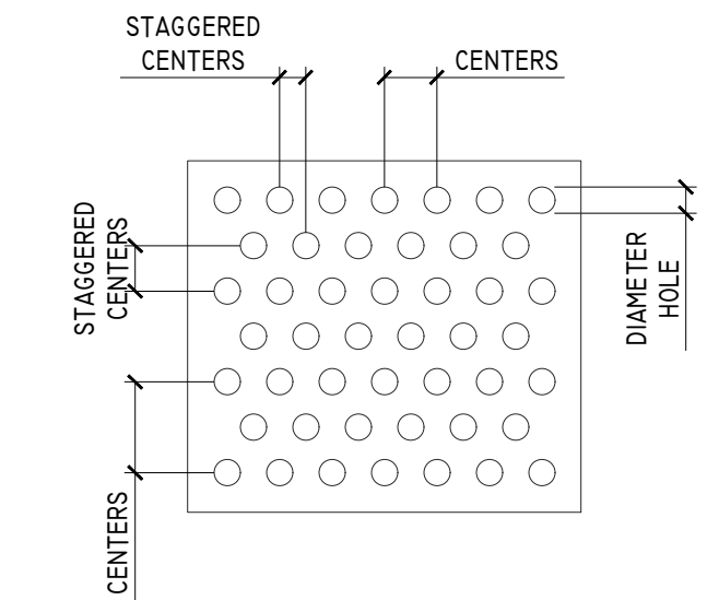
3 STAGGERED ROUND HOLES AI SCALE: 3"=1'-0"
